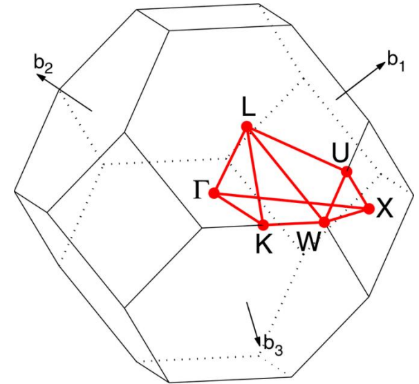
面心立方
