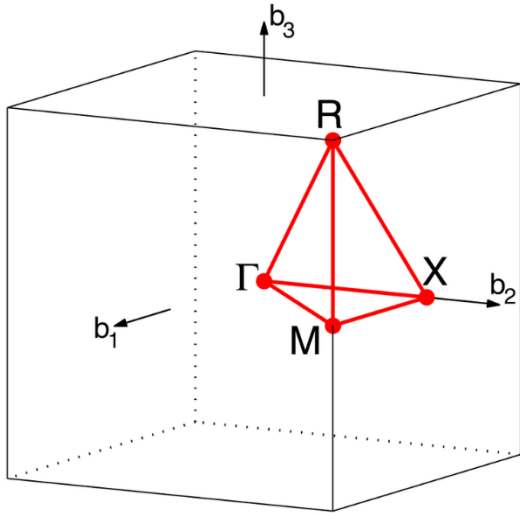
简单立方
